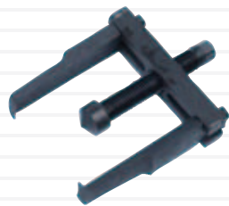
800-TA6702 兩爪薄型曲軸正時齒輪拉拔器 CRANKSHAFT TIMING GEAR PULLER
