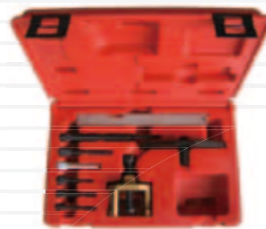
601-CSSC8076 福特/馬自達 正時工具組 ENGINE TIMING LOCKING TOOL SET-MAZDA & FORD
