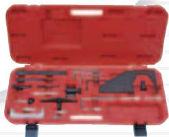
601-CSSC3156 馬自達、福特正時工具組 ENGINE TIMING TOOL SET- MAZDA and FORD
